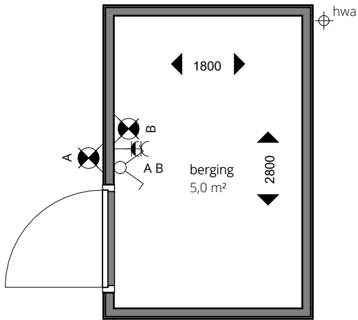
berging 1 : 50
