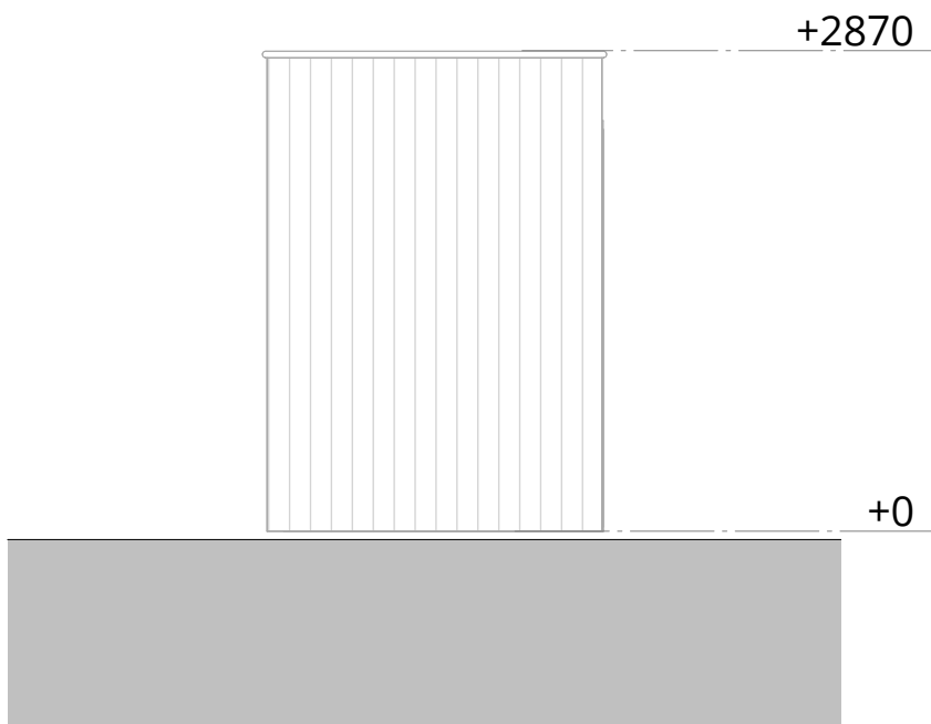
achtergevel 1 : 50
